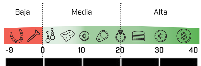
Posiciones de corte de tono (aproximadas) del VANQUISH 340.
